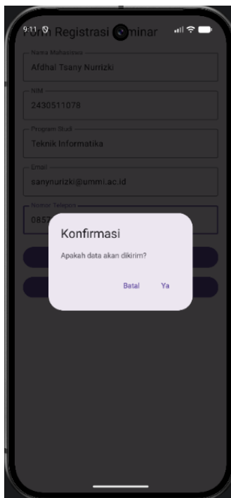
Gambar 3. Dialog Konfirmasi
